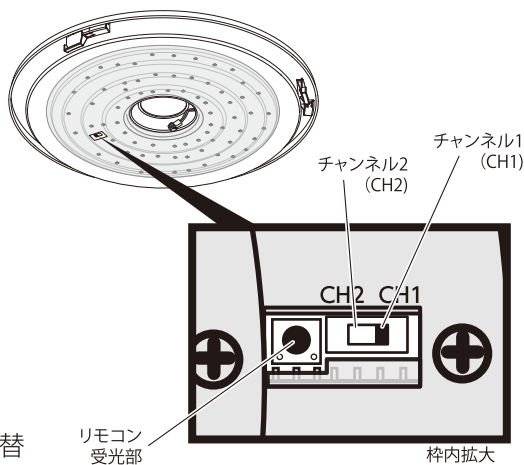
本体用チャンネル設定スイッチ
